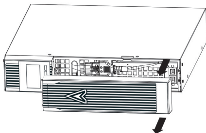
Рисунок 5. Извлечение передней панели ИБП
