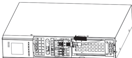
Рисунок 6. Подключение внутренних аккумуляторных батарей ИБП
