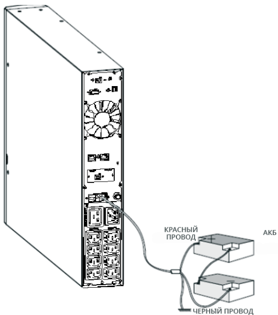
Рисунок 15. Подсоединение ВБМ
