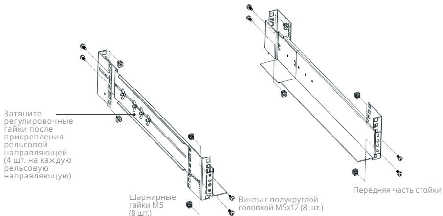
Рисунок 2. Крепление направляющих
