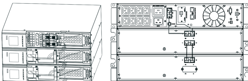
Рисунок 10. Стандартная установка ВБМ
