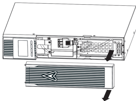
Рисунок 8. Снятие передней панели ВБМ
