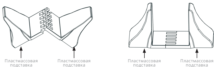
Рисунок 11. Установка пластмассовой подставки
