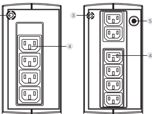
Рис. 2: Вид сзади
