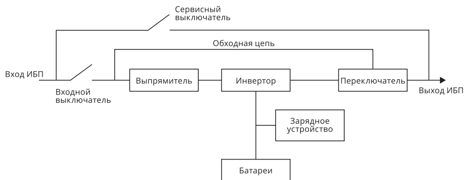
Рис. 1: Блок-схема ИБП
