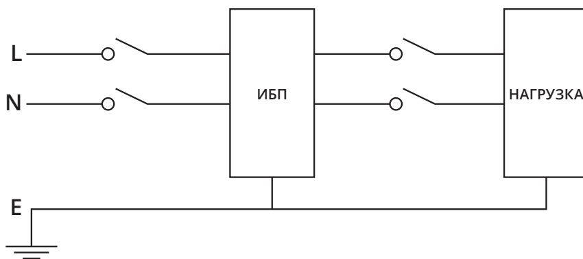
Рис. 23: Подключение кабелей
