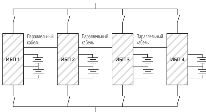
Рис. 25: Параллельная система
