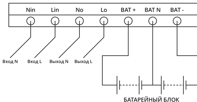
Рис. 24: Подключение к клеммной колодке
